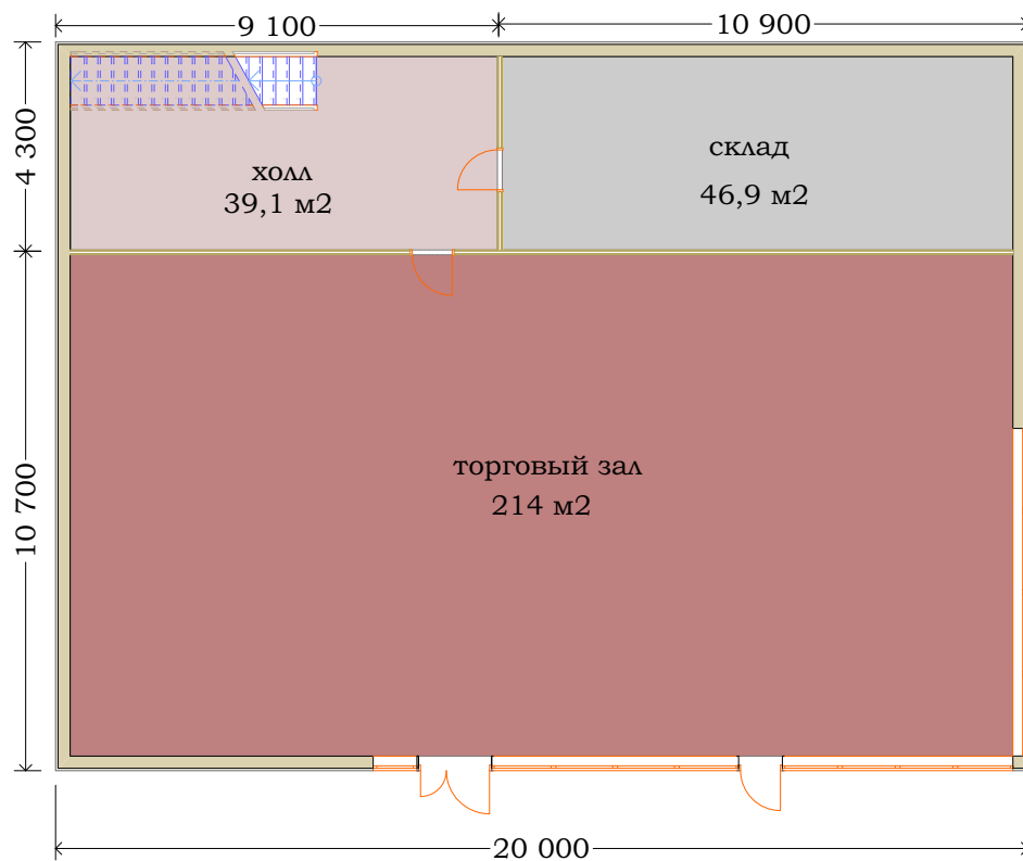
1 этаж
