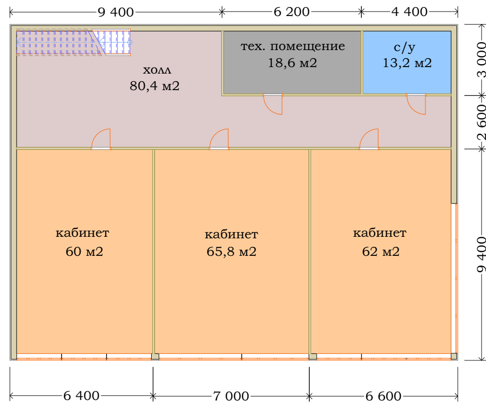
2 этаж
